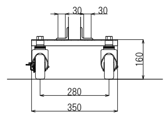
中間足 1/2
