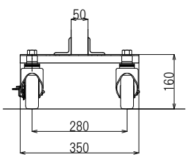
先頭柱 1/2
