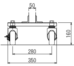
先端柱 1:2
