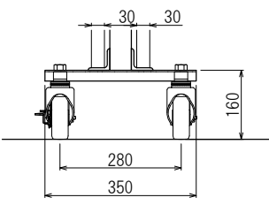
中間足 1:2
