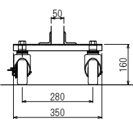
先頭柱 1:2
