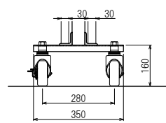
中間足 1:2
