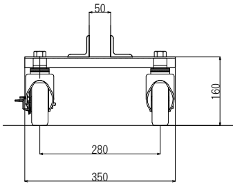
先頭柱 1:3
