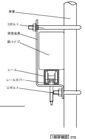
A部詳細図 1/2
