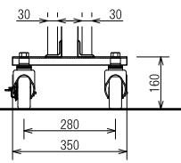
中間足 1:2
