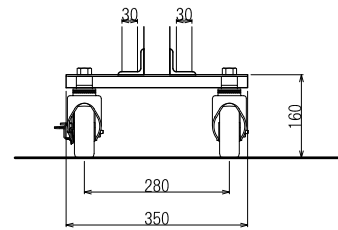
中間足 1:3
