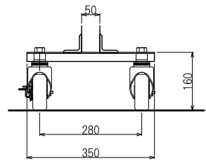
先頭柱 1:3
