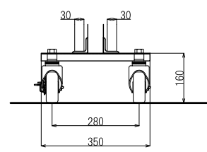
中間足 1:3
